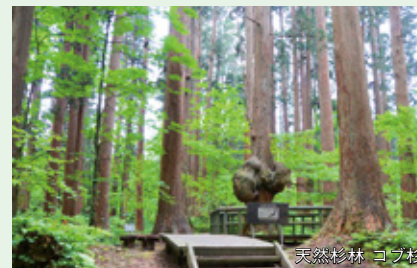
天然杉林 コブ杉
